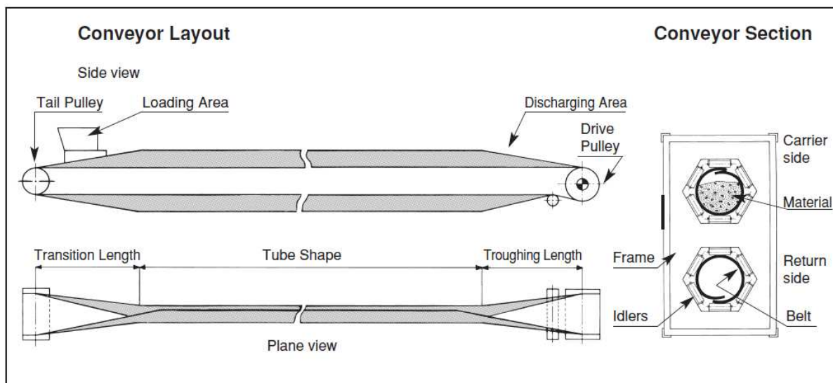
Figura 3.10 - Diagrama esquemático de funcionamento do Tube Belt Conveyor
