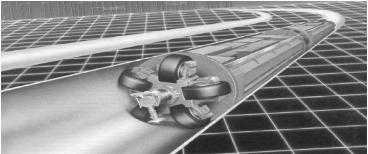
Figura 3.6 – Cápsula Pneumática em Duto – mineradora no Japão Fonte: Liu (2000)
