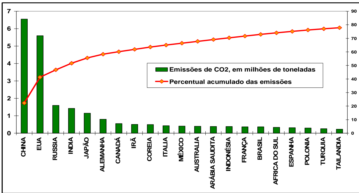
Figura 4.2 – Emissões por países e acumulada pelos grandes emissores Fonte: IEA (2010)
