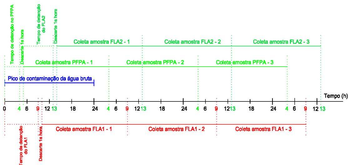
Figura 5.11: Esquema de coleta de amostra dos experimentos em que foi avaliado o traspasse.
