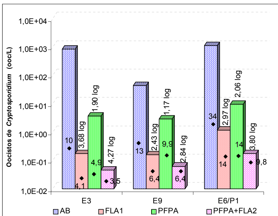
Figura 5.8: Valores de concentração de oocistos e turbidez nos experimentos sem amadurecimento e com taxa de filtração igual a 3 m 3 /m 2 .d.
