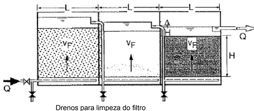
Figura 3.9: Esquema em corte de uma instalação de pré-filtração em pedregulho com escoamento ascendente em unidades em série – PFPAS (Wegelin, 1996)
