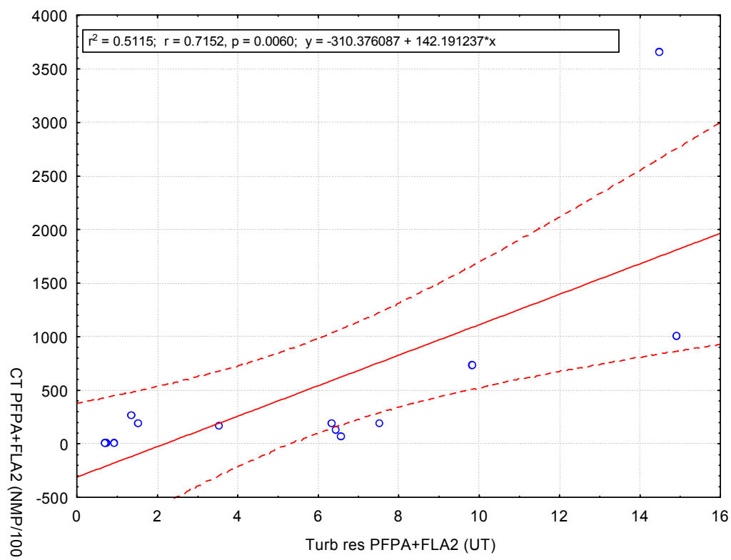
Figura 5.26: Associação entre concentração de coliformes totais e turbidez no efluente da sequência de tratamento PFPA+FLA2 (n=12).
