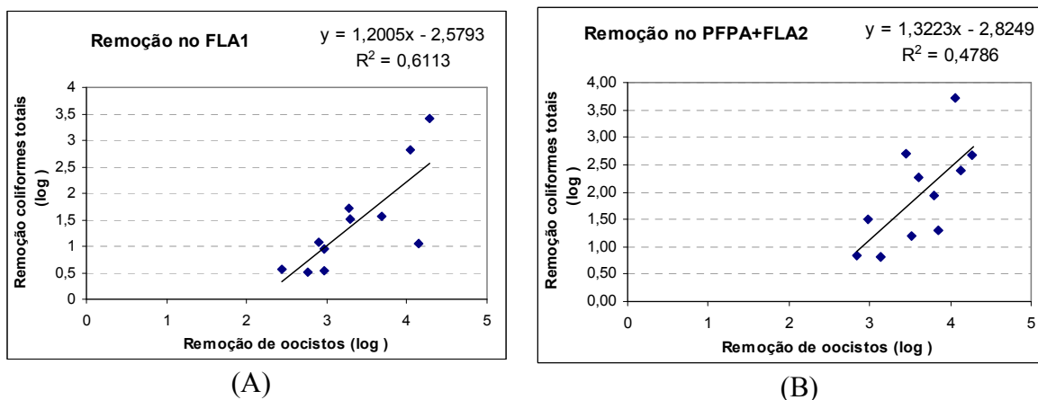
Figura 5.10: Associação entre valores de log – remoções de coliformes totais e de oocistos de Cryptosporidium , nas primeira e segunda fases, para as seqüências de tratamento (A) FLA1 e (B) PFPA+FLA2.
