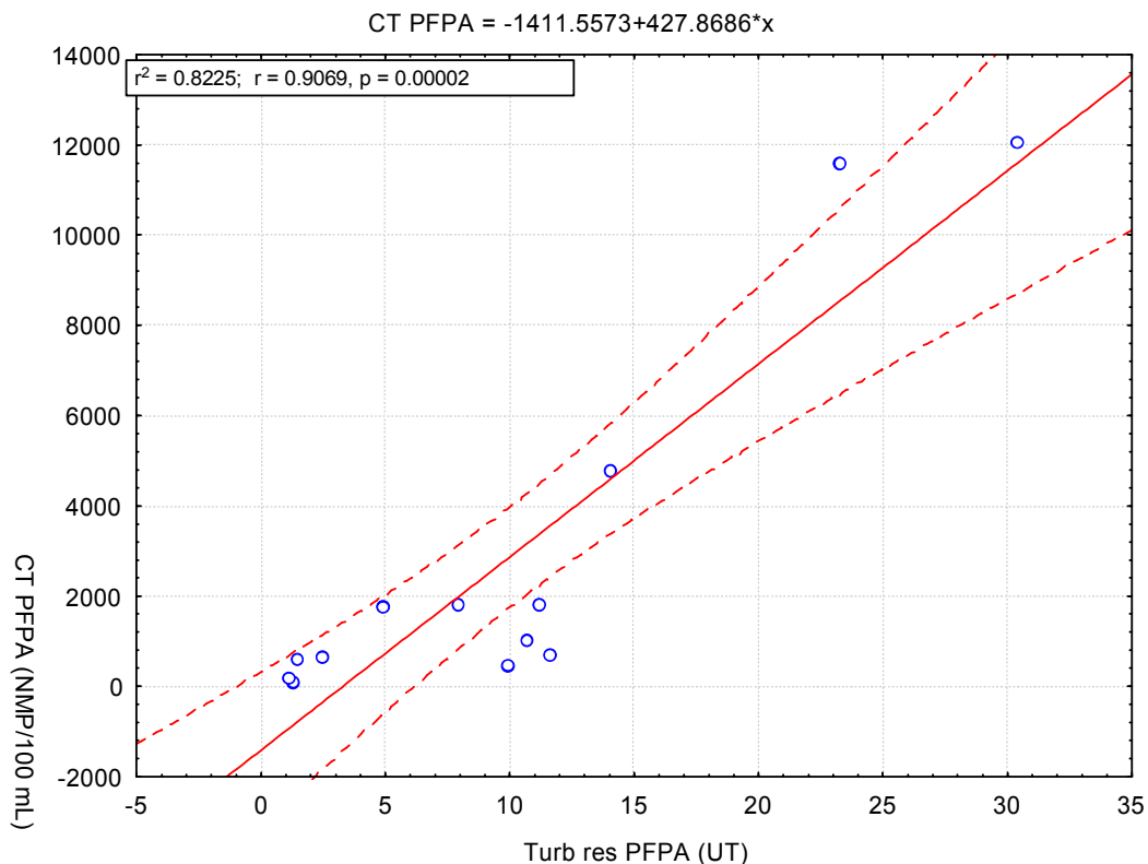
Figura 5.25: Associação entre valores de coliformes totais e turbidez residual no efluente do PFPA (n=13).
