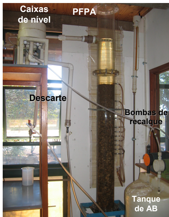
Figura 4.4: Instalação piloto do Pré-filtro de pedregulho com fluxo ascendente (PFPA)
