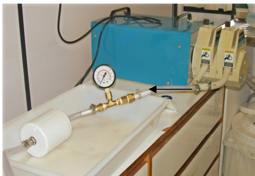
Figura E.1: Filtração com auxílio de bomba peristáltica
