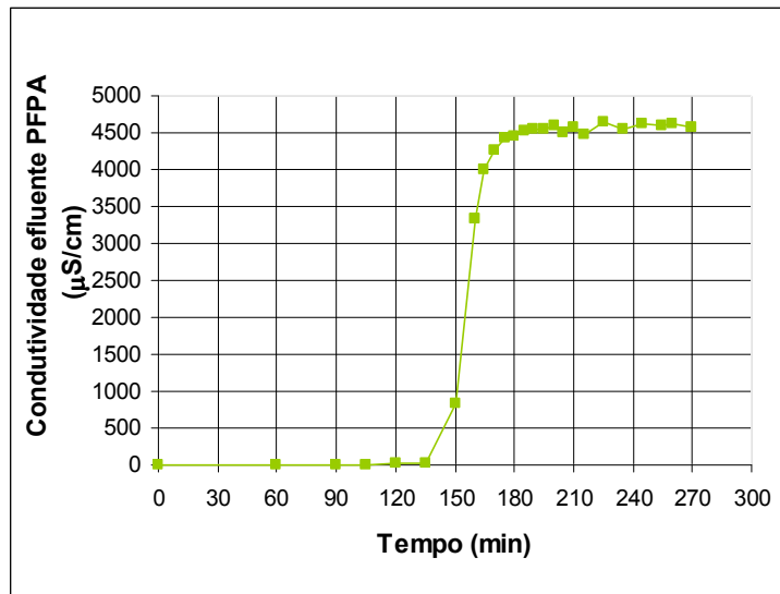
Figura 5.2: Curva da condutividade do teste com solução salina no PFPA para taxa de filtração de 10 m 3 /m 2 .d.
