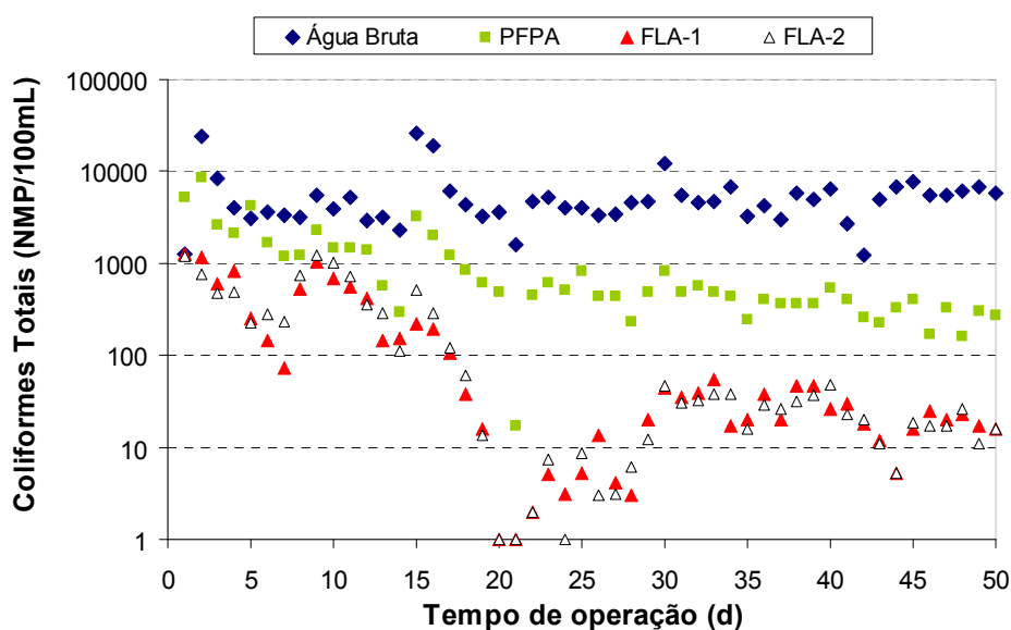
Figura 5.5: Comportamento de coliformes totais ao longo do tempo de operação das unidades de filtração durante os estudos preliminares.
