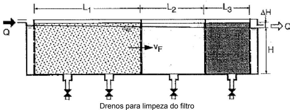
Figura 3.11: Esquema em corte de uma instalação de pré-filtração em pedregulhos com escoamento horizontal em câmaras em série (Wegelin, 1996)
