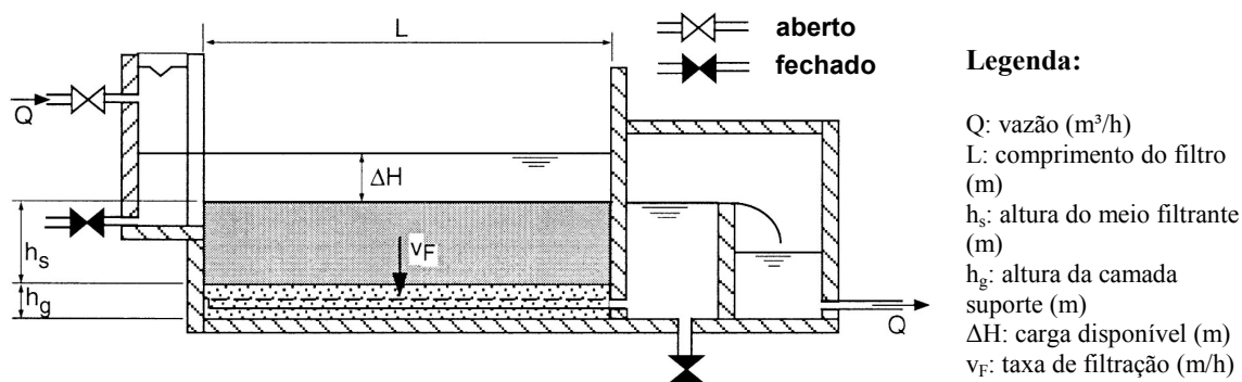
Figura 3.3: Esquema de um filtro lento (Wegelin 1996, modificado).
