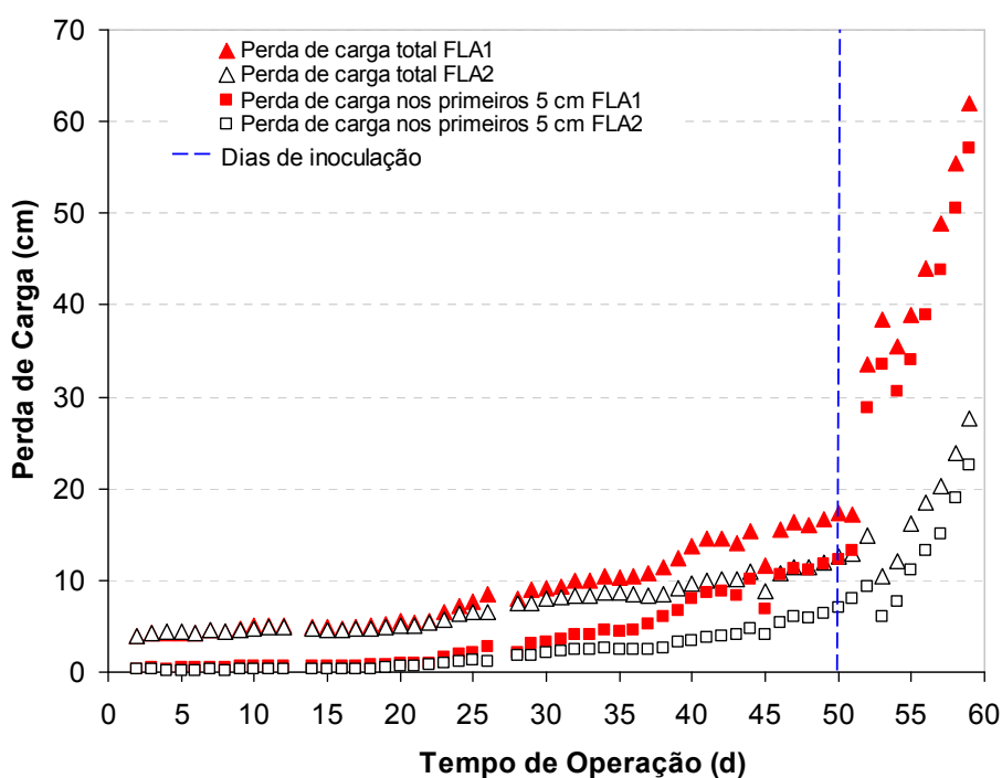
Figura 5.6: Evolução da perda de carga total e nos primeiros 5 cm dos filtros lentos durante os estudos preliminares.
