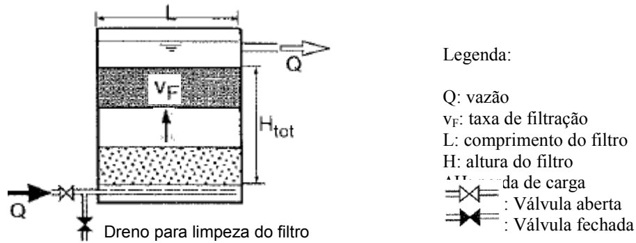
Figura 3.10: Esquema em corte de uma instalação de pré-filtração em pedregulhos com escoamento ascendente em camadas – PFPAC (Wegelin, 1996)
