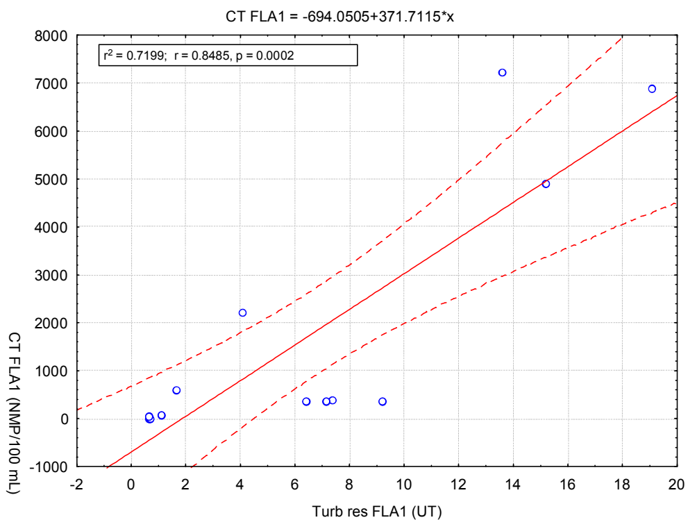
Figura 5.29: Associação entre concentração de coliformes totais e turbidez no efluente do FLA1. (n=13)
