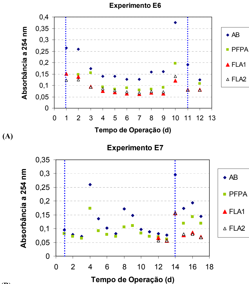
Figura 5.7: Comportamento dos valores de Absorbância a 254 nm nas unidades de filtração no (A) Experimento E6 e (B) Experimento E7.
