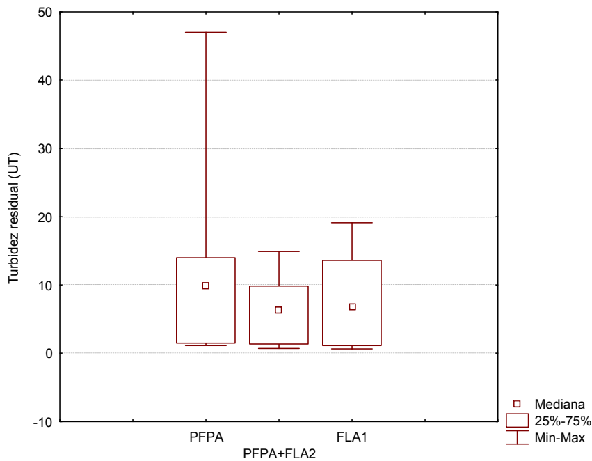
Figura 5.24: Turbidez dos efluentes de cada unidade de tratamento (para taxas de filtração dos filtros lentos iguais a 3 e 6 m/d).
