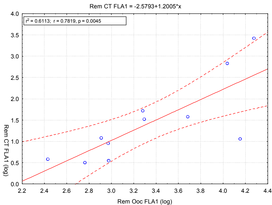
Figura 5.27: Associação entre remoção de coliformes totais e remoção de oocistos de Cryptosporidium pelo filtro lento sozinho, FLA1. (n=11)
