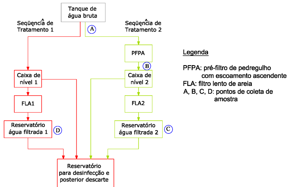
Figura 4.2: Fluxograma da instalação piloto.
