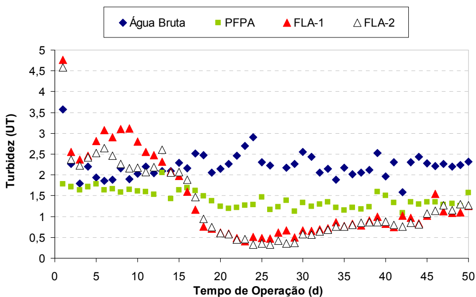
Figura 5.4: Comportamento da turbidez nas unidades de filtração nos primeiros 50 dias da primeira fase (estudo preliminar).
