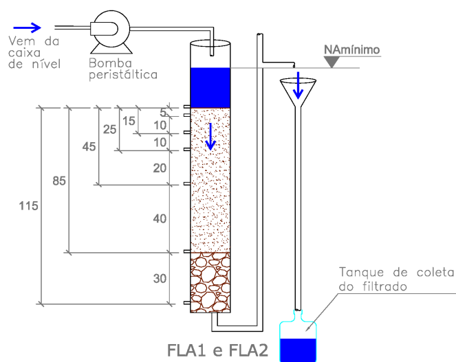
Figura 4.6: Detalhe das tomadas de pressão nos filtros lentos FLA1 e FLA2 para observação das perdas de carga nesses filtros..
