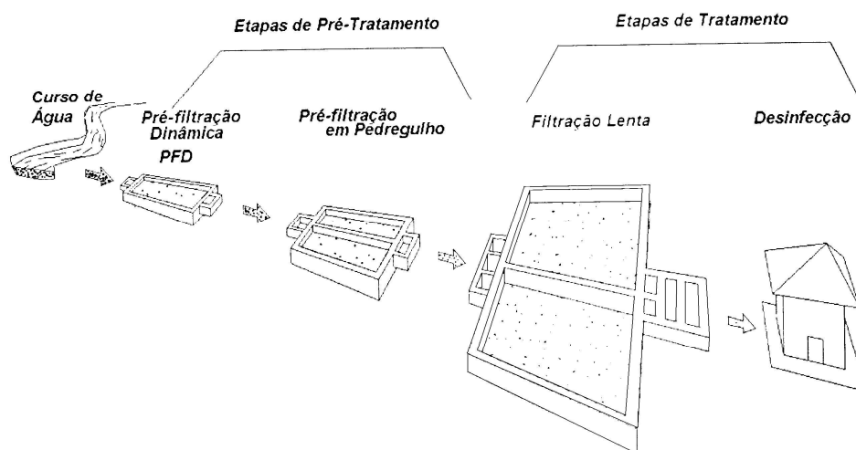
Figura 3.7: Esquema geral de uma instalação de filtração em múltiplas etapas - FIME (Di Bernardo e Dantas, 2005, modificado)
