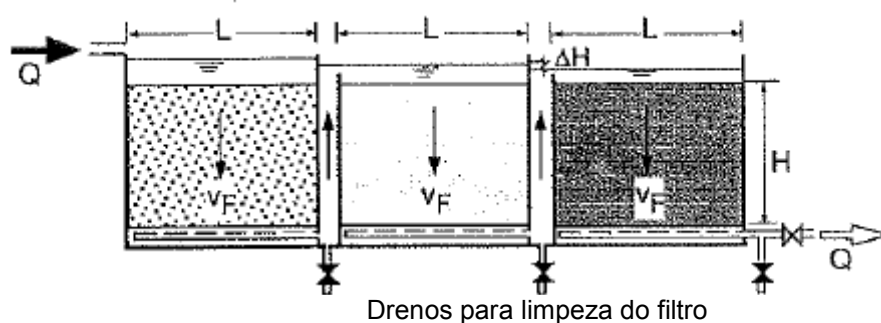
Figura 3.8: Esquema em corte de uma instalação de pré-filtração em pedregulho com escoamento descendente em unidades em série (Wegelin, 1996)
