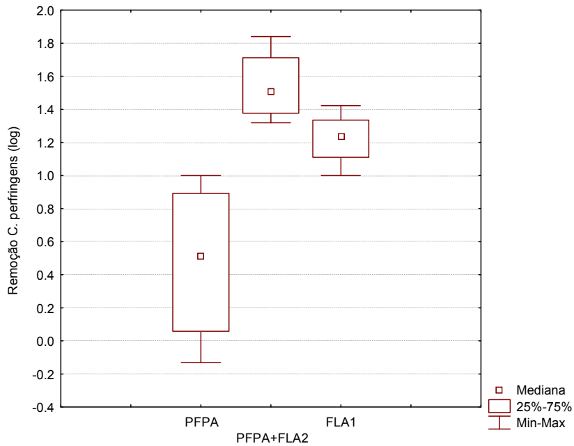
Figura 5.21: Remoção de Clostridium perfringens em cada unidade de tratamento (para taxa de filtração dos filtros lentos igual a 6 m/d).
