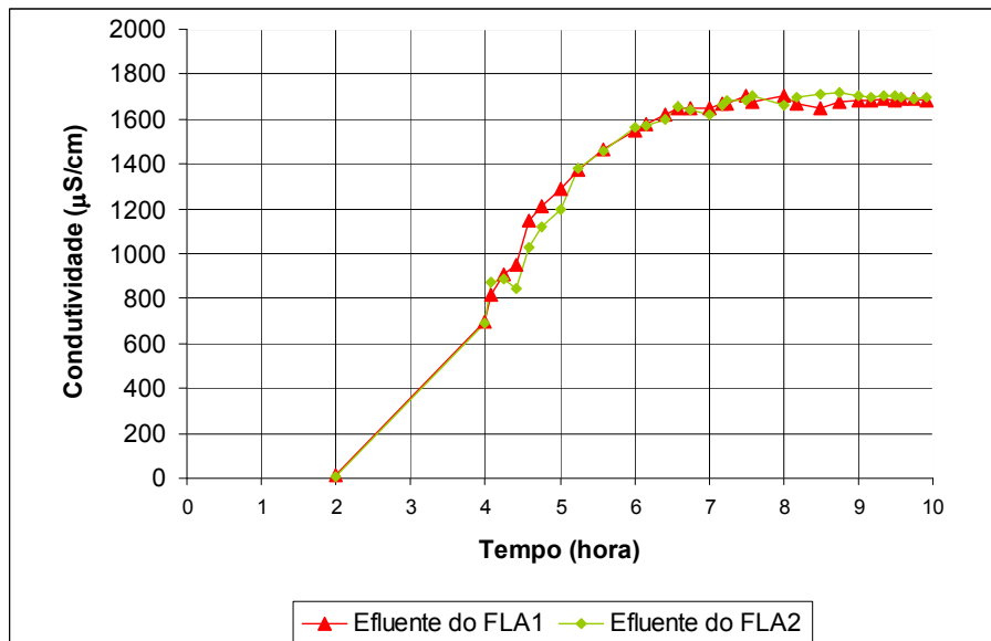
Figura 5.3: Curva da condutividade do teste com solução salina no FLA1 e FLA2 para taxa de filtração de 3 m 3 /m 2 .d.
