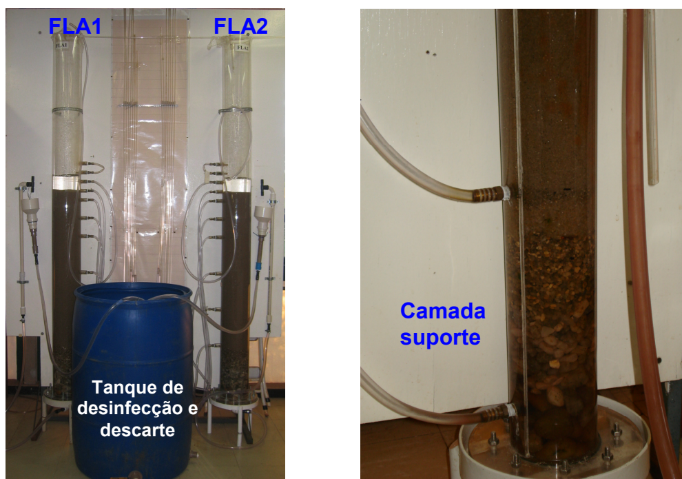
Figura 4.5: Instalação piloto dos Filtros lentos de areia (FLA1 e FLA2)
