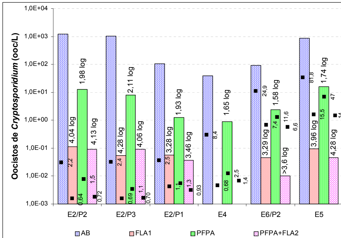
Figura 5.9: Valores de concentração de oocistos e turbidez nos experimentos em que os filtros lentos foram submetidos a algum período de amadurecimento e operados com taxa de filtração igual a 3 m 3 /m 2 .d.
