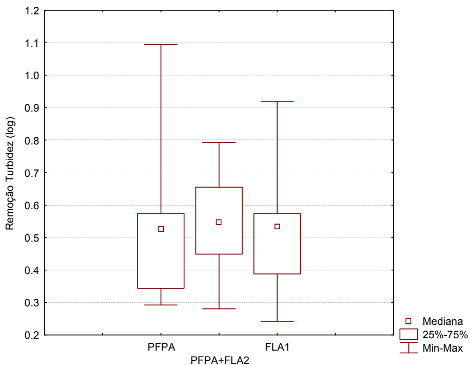
Figura 5.20: Remoção de turbidez em cada unidade de tratamento (para taxas de filtração dos filtros lentos iguais a 3 e 6 m/d).
