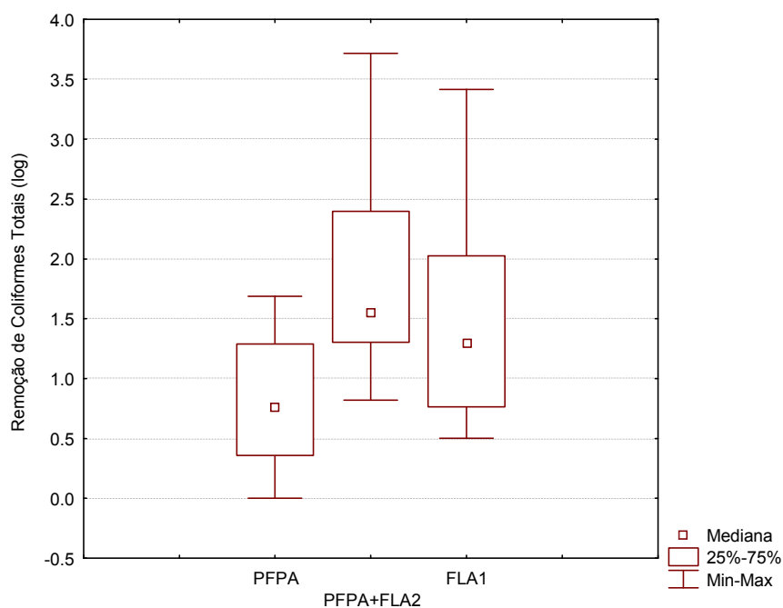
Figura 5.19: Remoção de coliformes totais em cada unidade de tratamento (para taxas de filtração iguais a 3 e 6 m/d).
