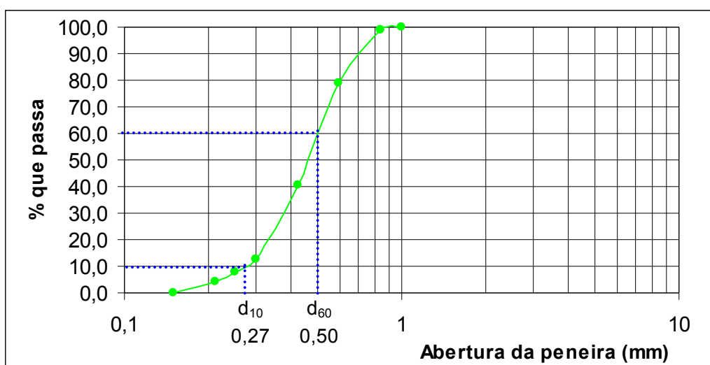
Figura 5.1: Curva granulométrica do meio filtrante dos filtros lentos FLA1 e FLA2.
