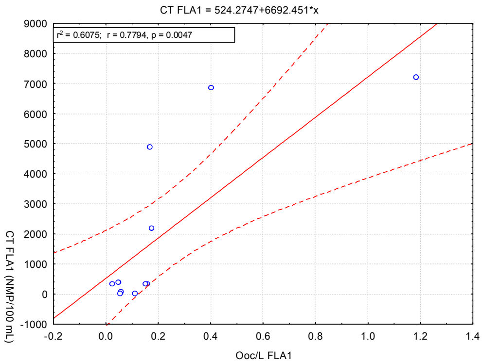
Figura 5.28: Associação entre concentração de coliformes totais e de oocistos de Cryptosporidium no efluente do FLA1. (n=11)
