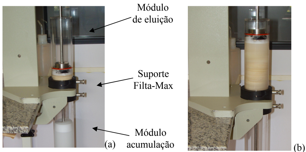
Figura E.3: Estação de eluição: (a) compressão; (b) descompressão
