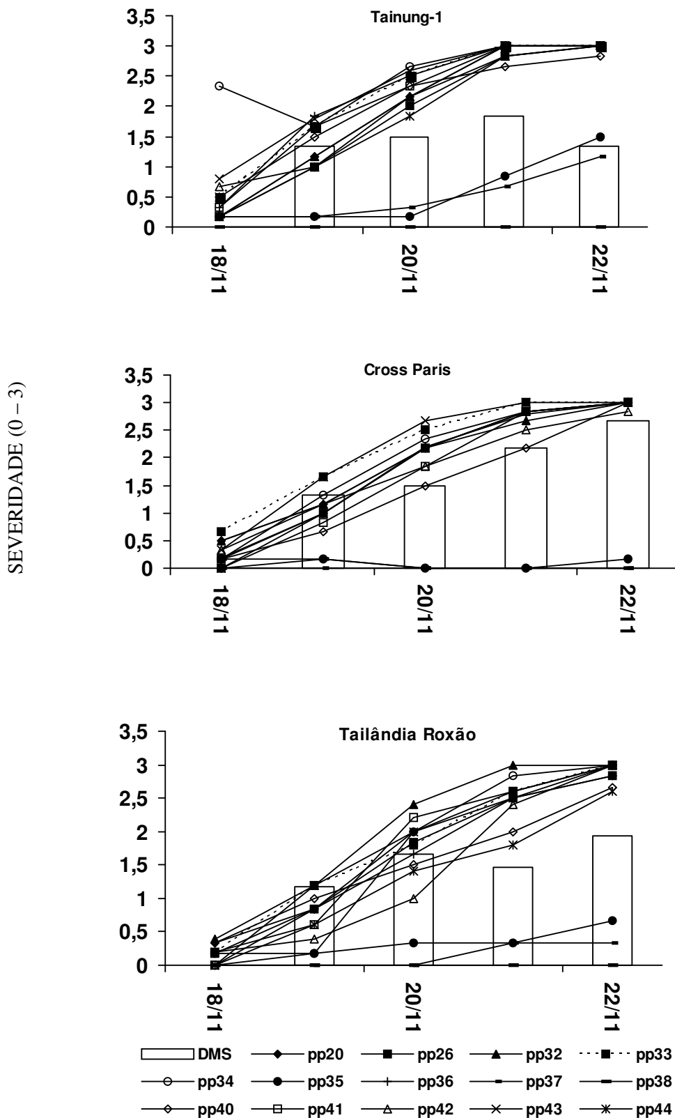
Fig. 7. Curvas representando o progresso da doença por 14 isolados de Phytophthora palmivora grupo III em três cultivares de mamão (Experimento II). DMS = diferença mínima significativa segundo o teste de Tukey ( p = 0,05 ); pp37 = isolado de pupunha; pp38 = isolado de Morremia odorata ; demais isolados foram retirados de frutos e raízes de mamoeiro.
