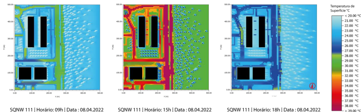
Figura 6 - Resultado da simulação às 09h, 15h e 16h.
