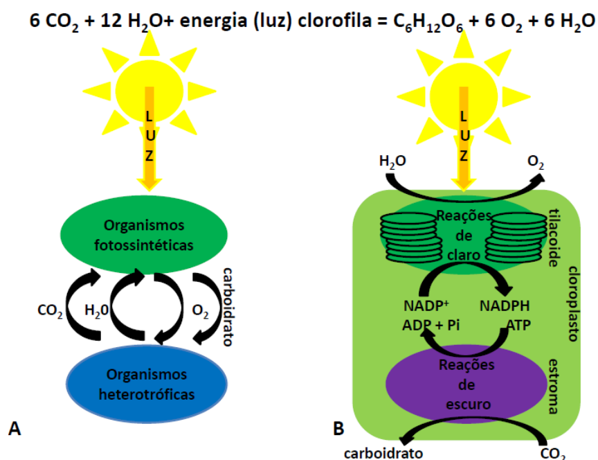
Figura 1. (A) A energia solar serve como uma fonte poderosa de toda a energia química e biológica. Os organismos fotossintéticos utilizam a energia da luz para produzir carboidratos e para liberação do \text{O}_2 pela fotólise de água, os quais vão ser utilizados por organismos heterotróficos. (B) As reações luminosas da fotossíntese geram NADPH (nicotinamida adenina dinucleótido fosfato) e ATP (adenosina trifosfato) ricos em energia e produzem oxigênio, gás mantido na atmosfera, às custas da energia solar. As moléculas NADPH e ATP produzidas nas reações de claro são usadas nas reações de assimilação de carbono, que ocorrem na fase de escuro, para reduzir o \text{CO}_2 e formar carboidrato. Adaptada de Nelson e Cox (2011, p. 742-743).
