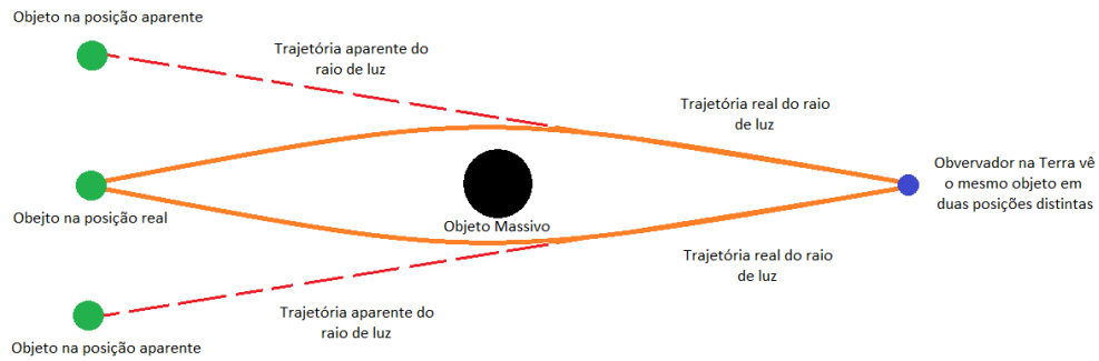
Figura 24 – Esquema simplificado da formação de múltiplas imagens por uma lente gravitacional.
