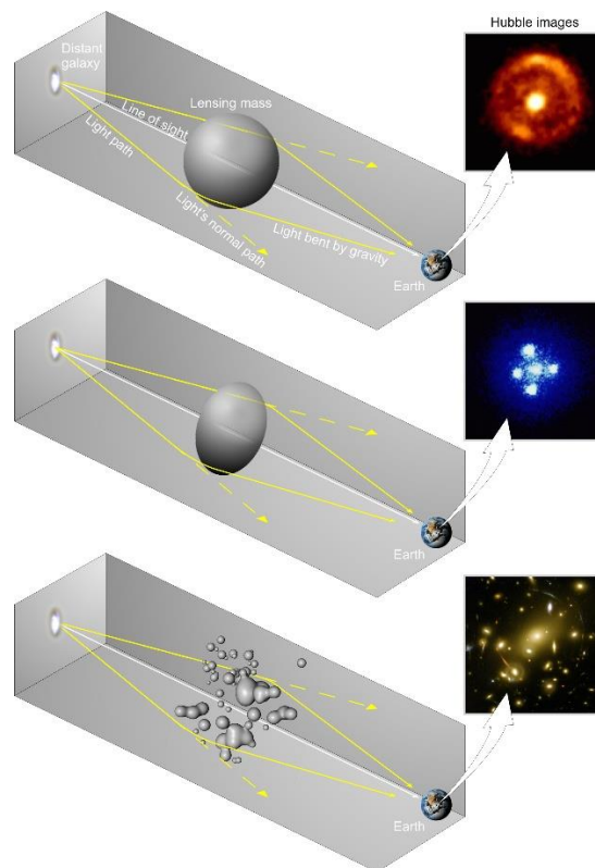
Figura 7 – Esquemas de Lentes Gravitacionais.
