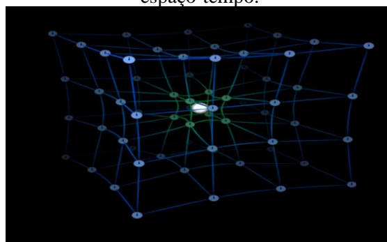
Figura 14 – Modelo 3D da deformação do espaço-tempo.
