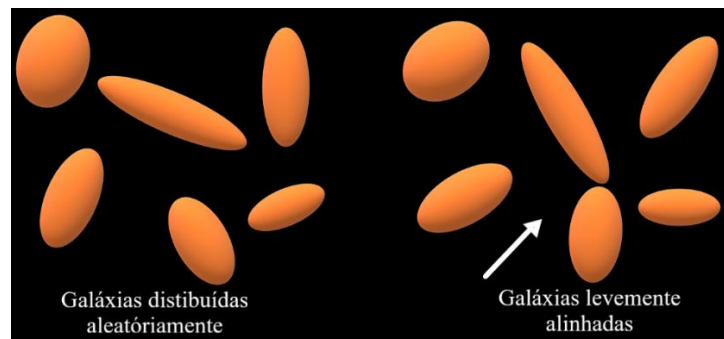
Figura 27 – Esquema simplificado de lente gravitacional fraca.
