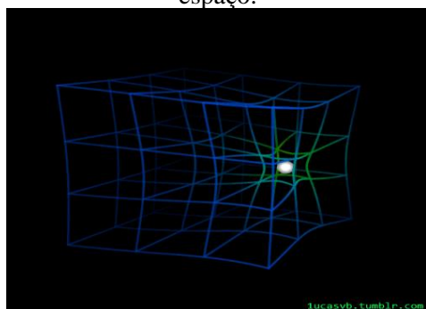
Figura 13 – Modelo 3D da deformação do espaço.
