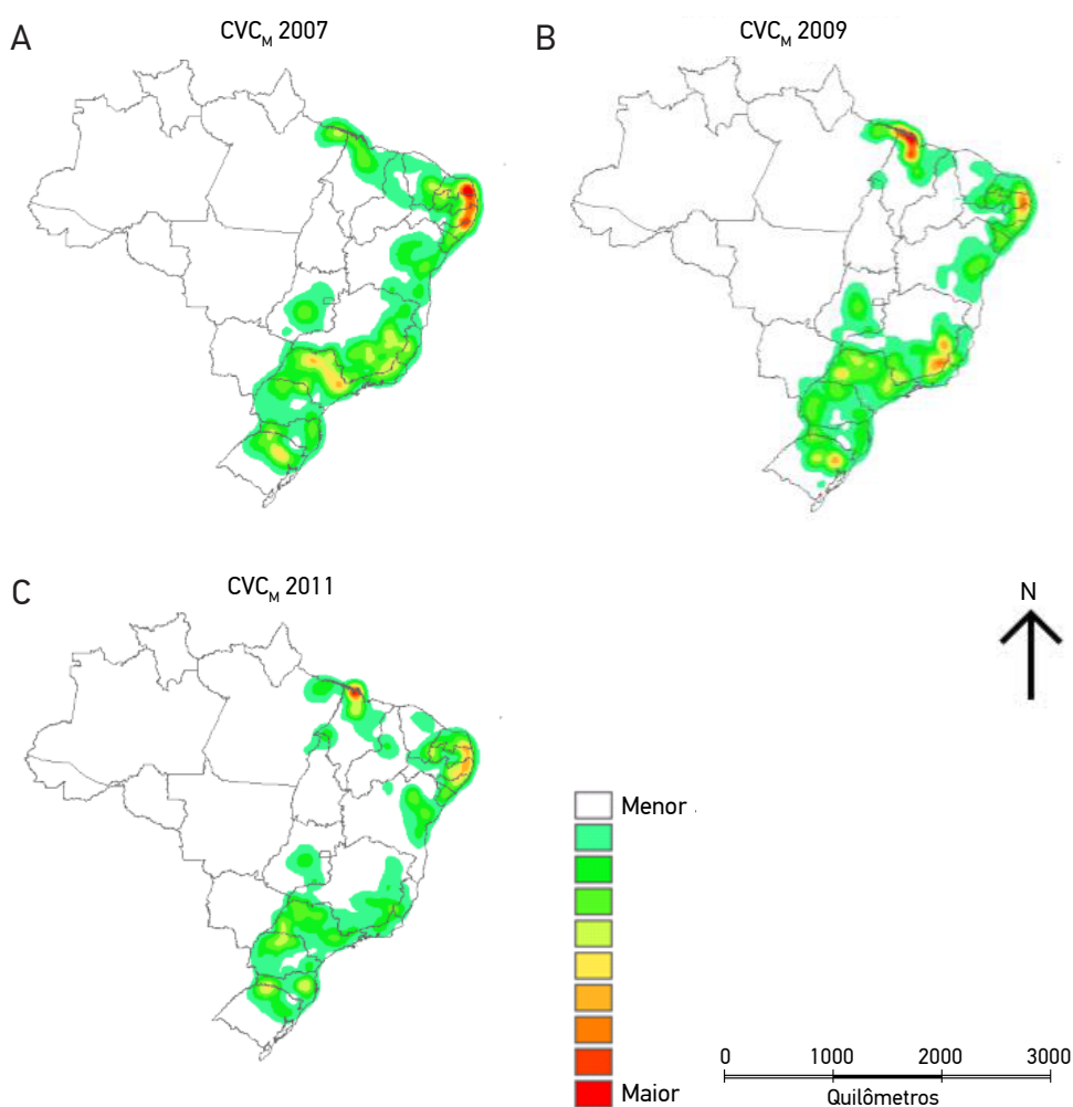
Figura 1. Superfície de densidade da Carga Viral Comunitária Média ( CVC_M ) dos indivíduos com AIDS de 13 anos de idade ou mais, monitorados pelos sistemas de vigilância do Brasil, método Kernel (atribuindo 50 cópias/ mL para os indivíduos com Carga Viral indetectável). Brasil, (A) 2007, (B) 2009 e (C) 2011.
