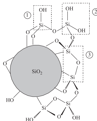
Figura 1. Esquema da estrutura da sílica gel. Em destaque os grupos silanol geminal (1), silanol vicinal (2) e siloxano (3)
