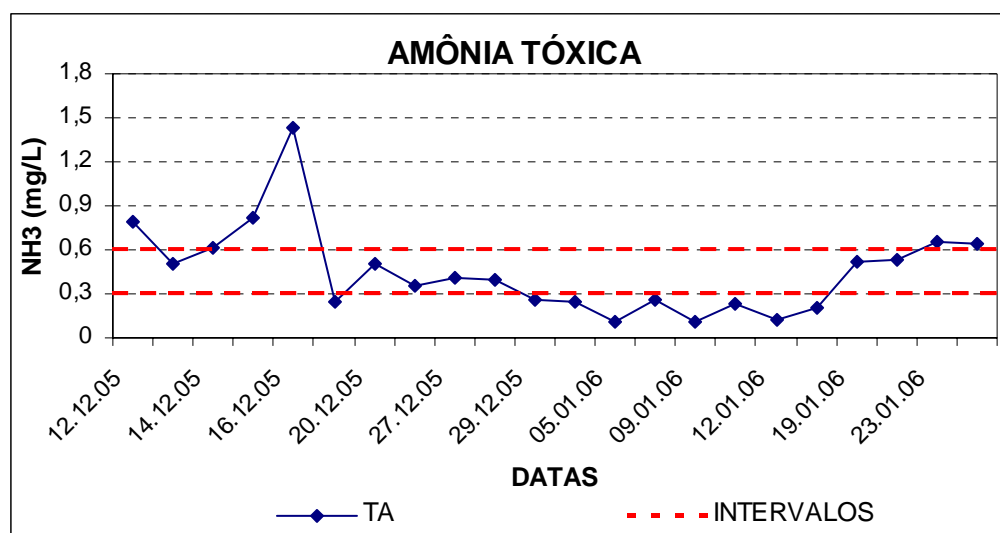
Figura 5.6: Concentração de amônia tóxica (NH 3 ) no tanque TA no decorrer do experimento 2.
