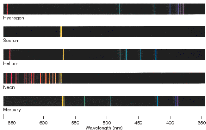
Figura 4 – Linhas de emissão dos elementos químicos H, Na, He, Ne, Hg
