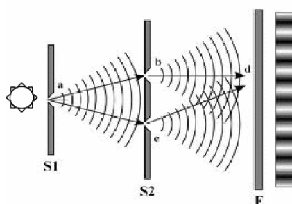
Figura 1 - Experimento da dupla fenda
