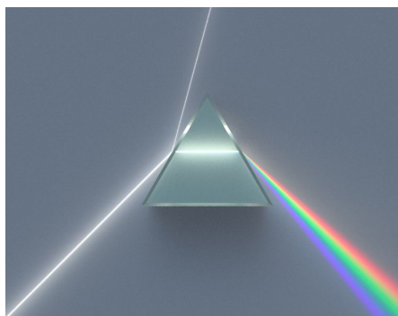
Figura 3 – Dispersão da luz solar
