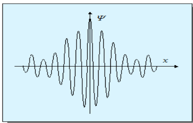
Figura 2 – Pacote de onda
