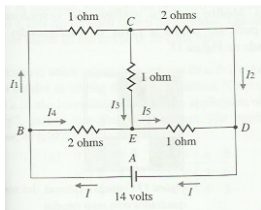
Figura 19: Circuito elétrico
