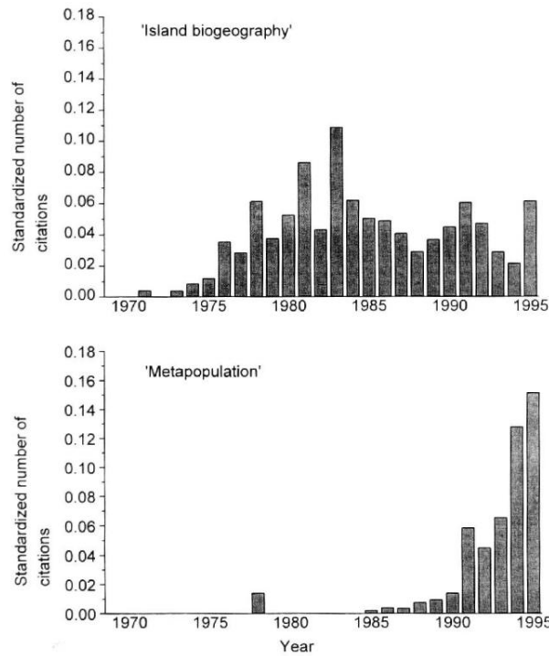
Figura 02. Histórico das citações de metapopulações e biogeografia de ilhas (Hanski & Simberloff, 1997).
