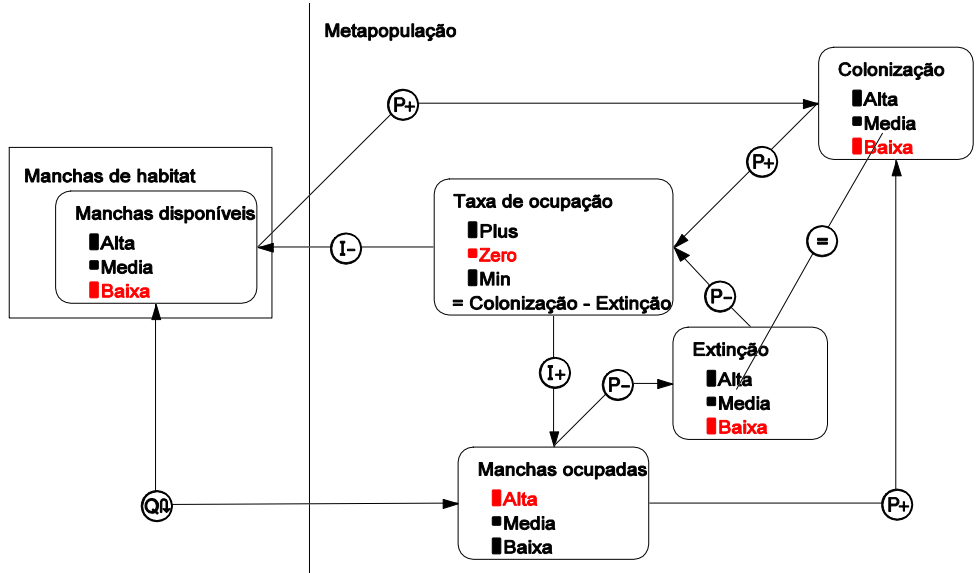
Figura 14. Modelo causal para o estado [38] da simulação do Cenário02 'Influência de fenômenos estocásticos de extinção e de colonização no crescimento de uma metapopulação'.
