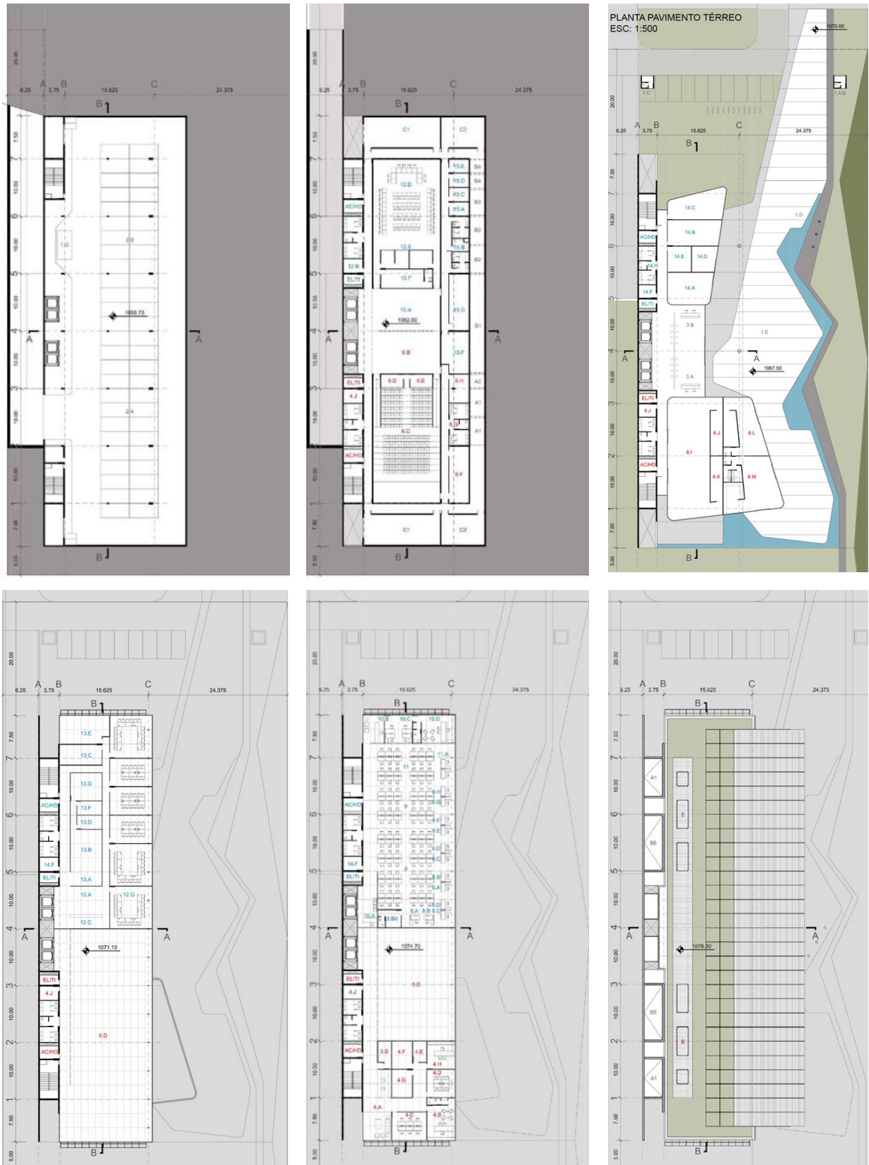
Figura 109. Plantas da proposta vencedora do concurso público nacional de projeto para a sede conjunta do CAU-BR e IAB-DF. A partir da imagem do canto superior esquerdo, em sentido horário: 2º subsolo, 1º subsolo, térreo, 1º pavimento, 2º pavimento e cobertura. Equipe coordenada pela arquiteta e urbanista Tais Cristina da Silva, São Paulo Arquitetos, 2016. Fonte: Acervo IAB DF.
