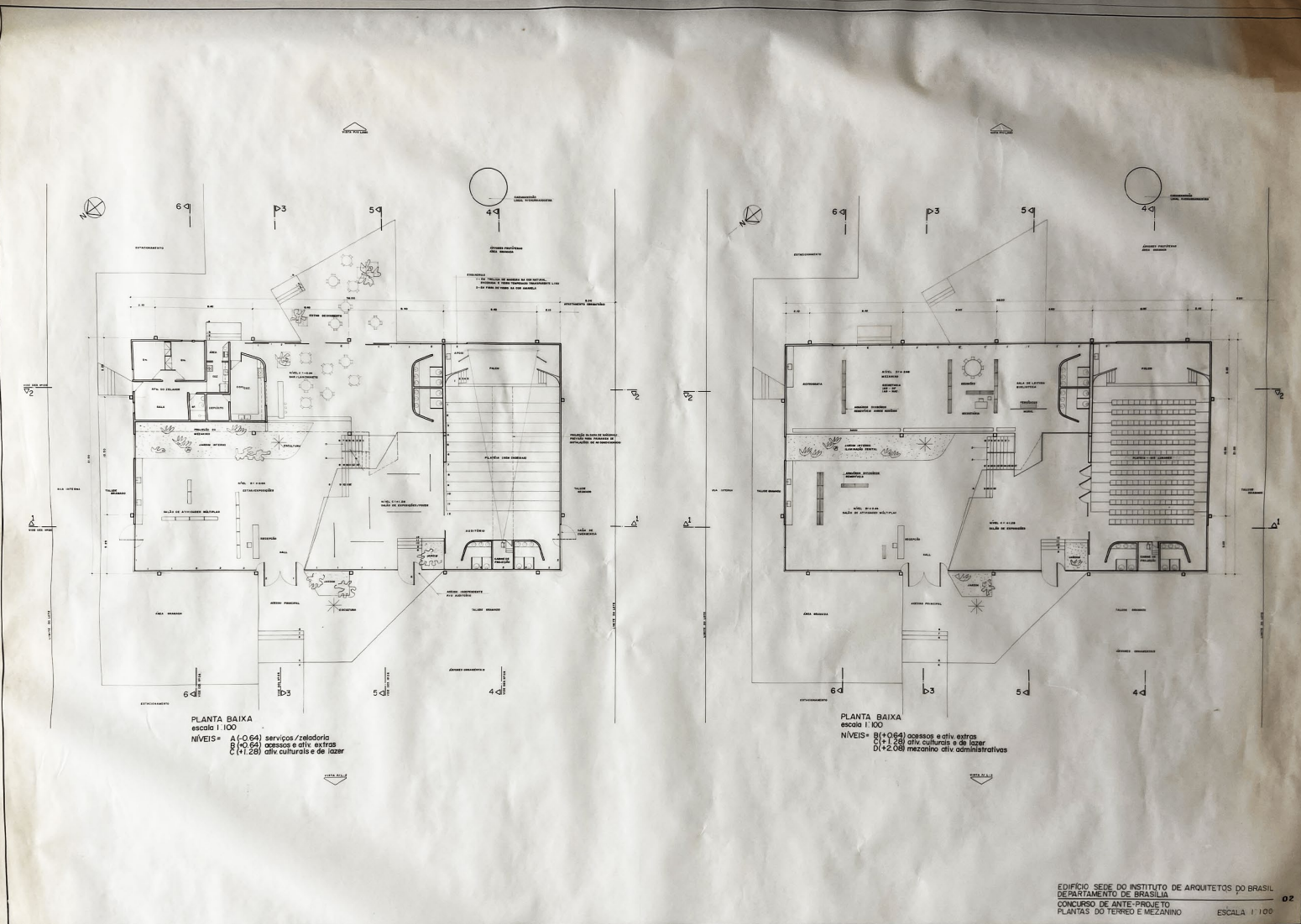
Figura 93. Prancha original apresentada no concurso de projeto para a Sede IAB DF. Plantas. Aleixo Furtado, 1979. Foto do autor. Fonte: Acervo IAB Brasília, Fundo IAB-DF.
