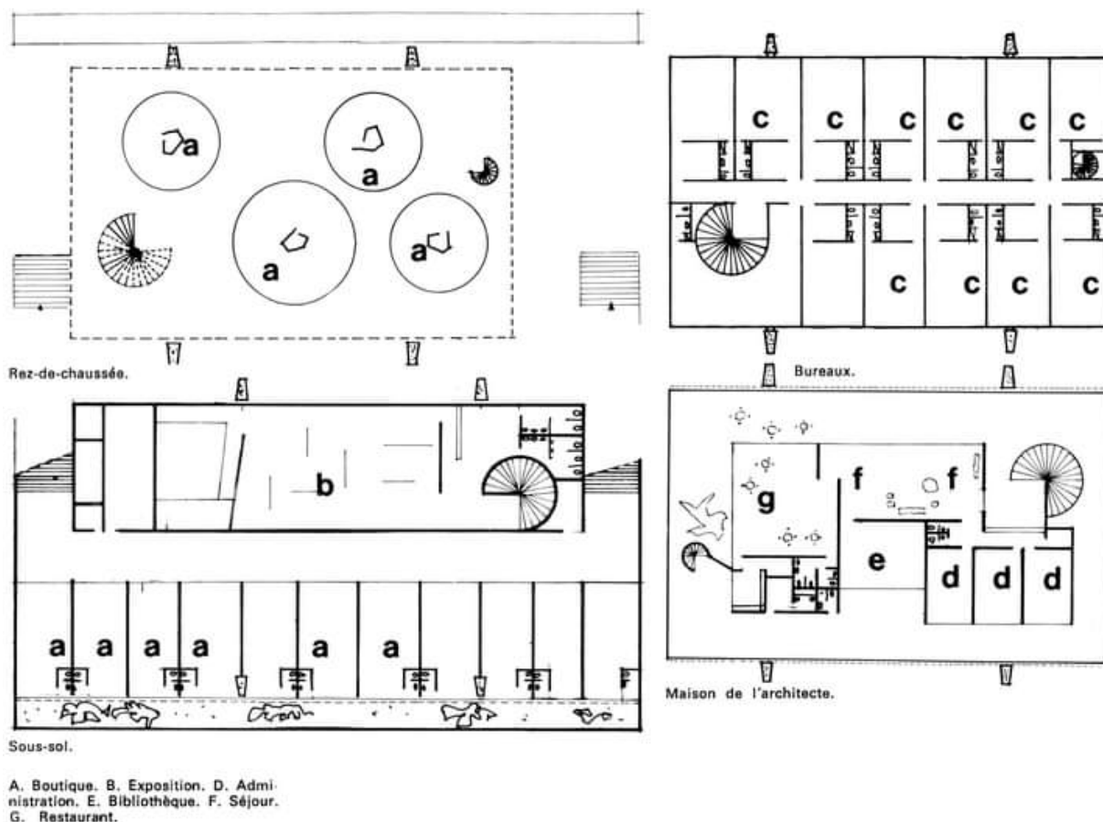
Figura 69. Plantas do projeto de Oscar Niemeyer para o IAB em Brasília publicadas na edição especial Oscar Niemeyer da revista L'Architecture d'aujourd'hui nº. 171, de 1974. Em sentido horário a partir do canto superior esquerdo: pilotis com lojas, primeiro pavimento destinado a escritórios, segundo pavimento, sede do IAB, IAB-DF e restaurante ("A casa dos arquitetos") e subsolo com auditório, sala de exposições e lojas. Fonte: Acervo IAB-DF.
