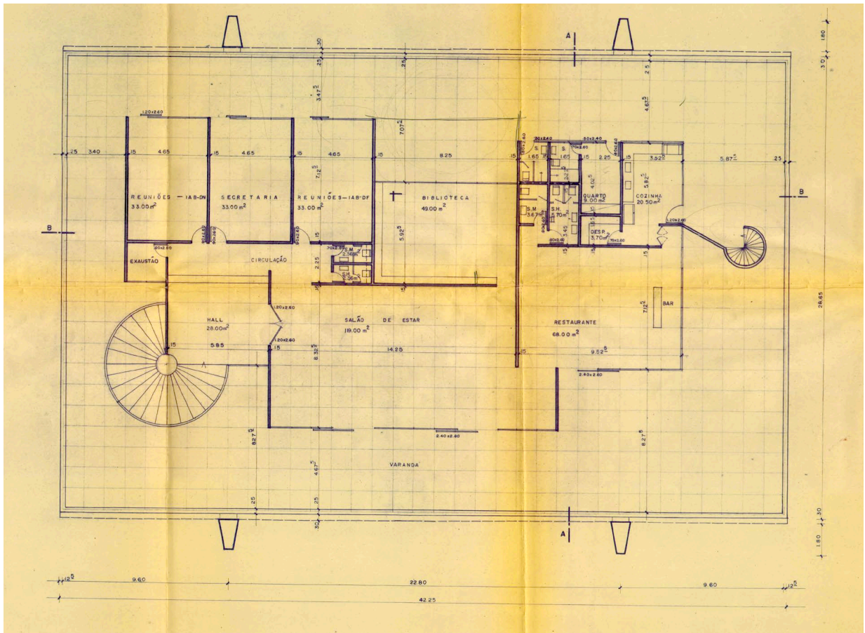
Figura 71. Prancha do 2º pavimento, ou pavimento de cobertura, do projeto de Oscar Niemeyer para o IAB. O espaço foi planejado para receber a sala de reuniões da Direção Nacional do IAB e a sala de reuniões do IAB-DF, entre elas há a secretaria, que seria compartilhada pelas duas instâncias. Há ainda biblioteca e restaurante além de ampla varanda coberta circundando todo o pavimento. Fonte: Acervo IAB Brasília, Fundo IAB-DF.
