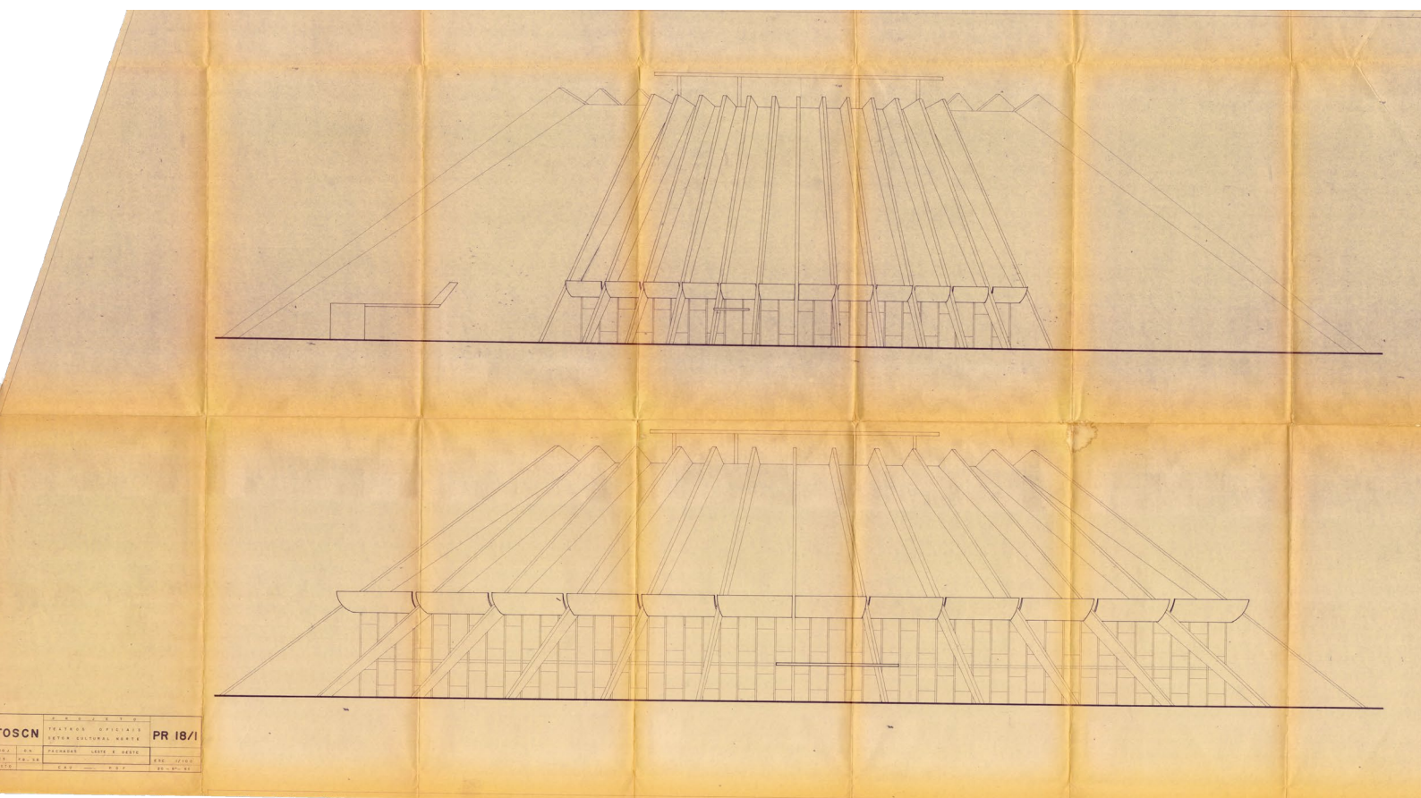
Figura 62. Corte longitudinal do Teatro Nacional Cláudio Santoro, de junho de 1966. De acordo com registros encontrados, o IAB-DF funcionou no pavimento imediatamente abaixo do terraço da cobertura. Fonte: Acervo IAB Brasília, Fundo IAB-DF.
