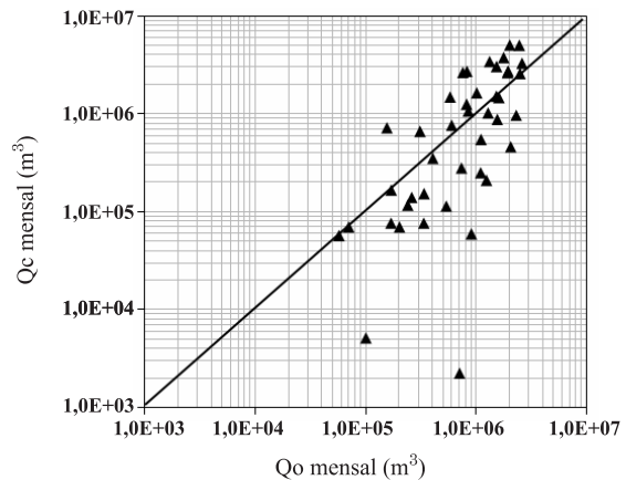
Figura 8. Valores mensais do volume de escoamento direto observados e calculados na bacia do ribeirão Pípiripau, no período de validação.
