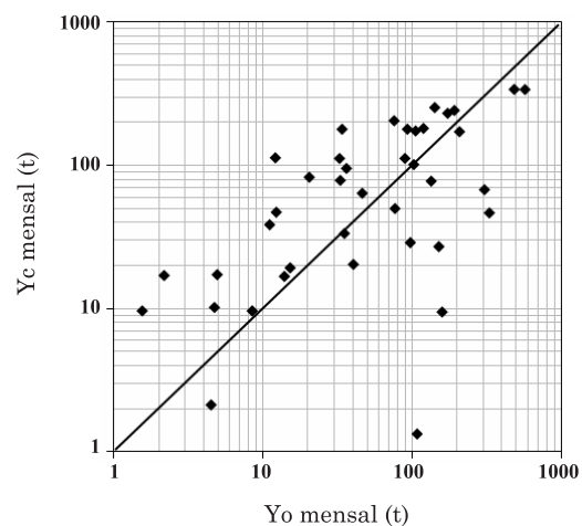
Figura 9. Valores mensais de aporte de sedimento observados e calculados na bacia do ribeirão Pípiripau, no período de validação.
