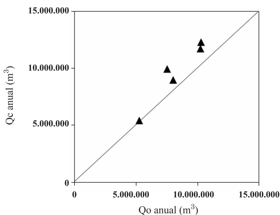
Figura 6. Valores anuais de escoamento direto observados e calculados pela equação 2 na bacia do ribeirão Pípiripau, no período de validação.
