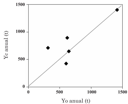
Figura 7. Valores de aporte de sedimento anual observados e calculados pela MUSLE modificada na bacia do ribeirão Pípiripau, no período de validação.
