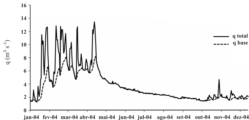
Figura 3. Decomposição do hidrograma em vazão total e escoamento de base para o ano de 2004, após a passagem do filtro digital.
